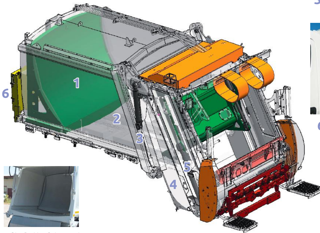
2 Glattflächige Seitenwände Kiefförmige Bodengruppe mit seitlichen Führungen für das Ausstoßschild.
